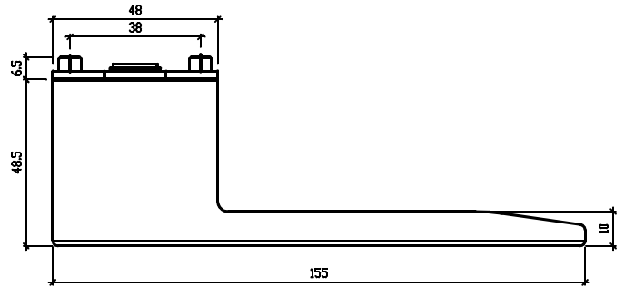
Widok z góry klamka I
