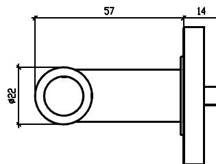
Widok z prawej strony klamka I
